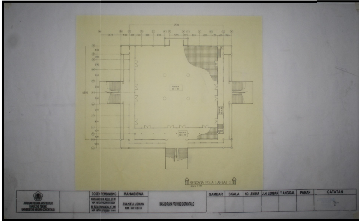
RENCANA POLA LANTAI 2
